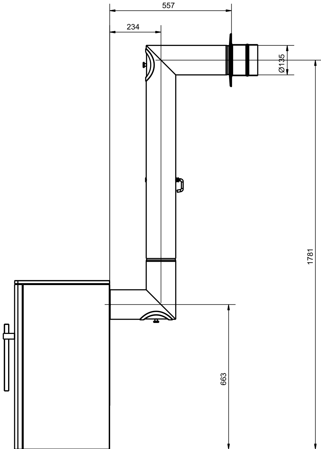
Iron-Dog 05 Rauchrohr vertikal
